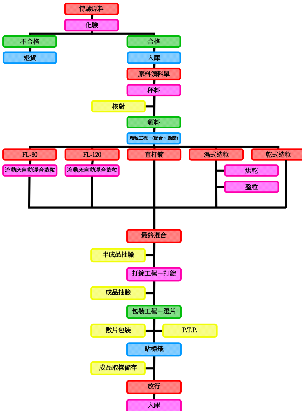
《錠劑製造流程圖》
